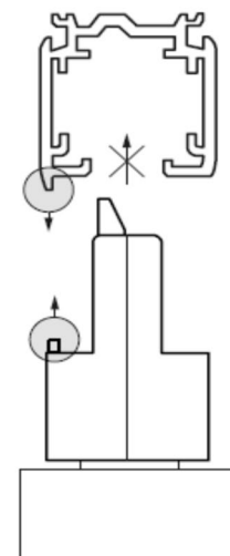
Неправильная установка
